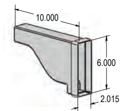
2" x 6" Scroll Pergola End
