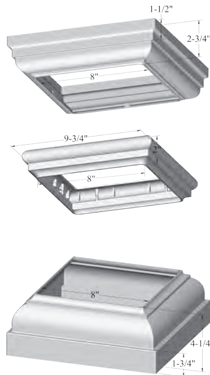
Trim Set
