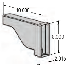
2" x 8" Scroll Pergola End
