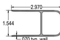
Light Alum. A-Channel
