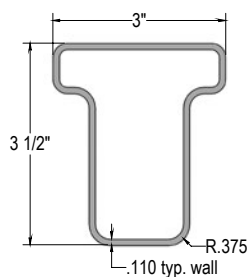
T-Rail
