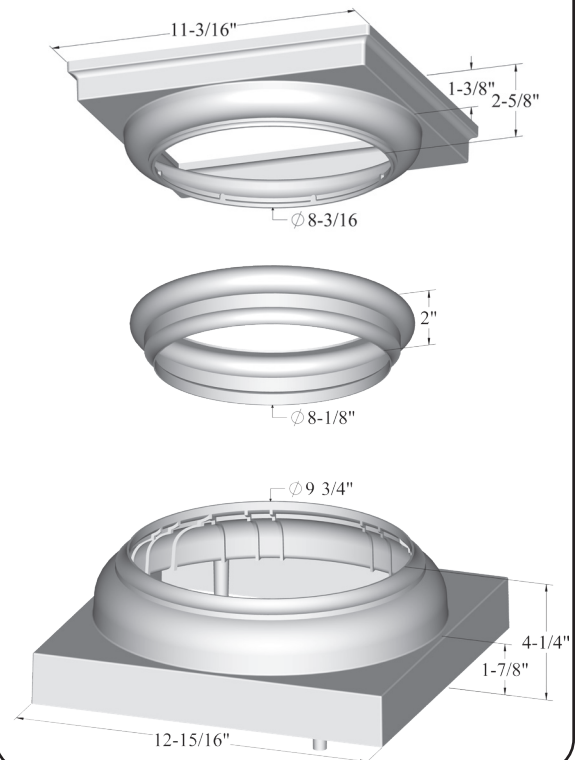
Trim Set
