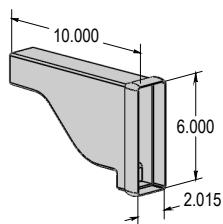
2" x 6" Scroll Pergola End
