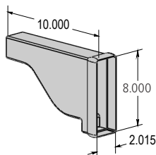
2" x 8" Scroll Pergola End
