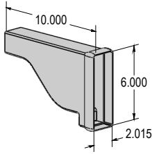
2" x 6" Scroll Pergola End
